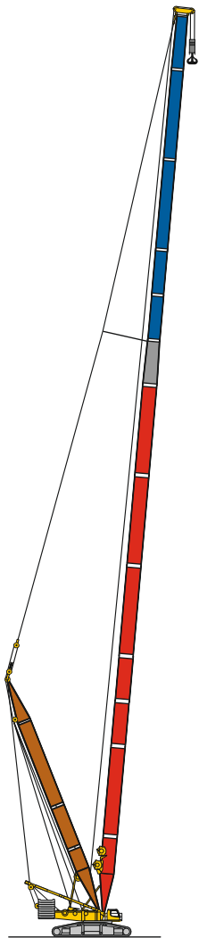
HSLD3 HSLD3B/BW HSL 56 m - 140 m D3 38,5 m
